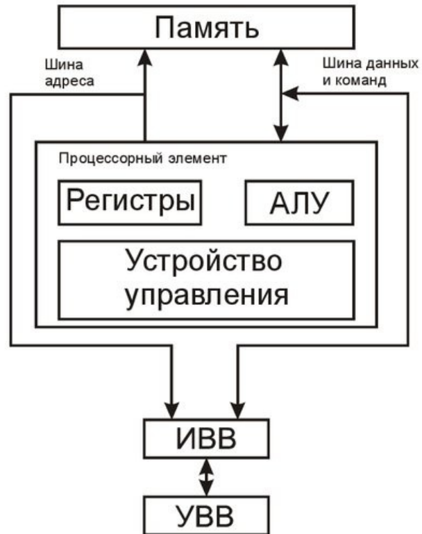
фоннеймановская архитектура
